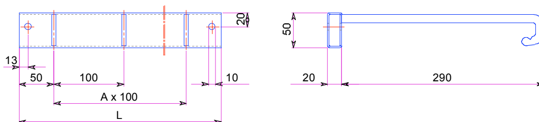
Frontansicht
